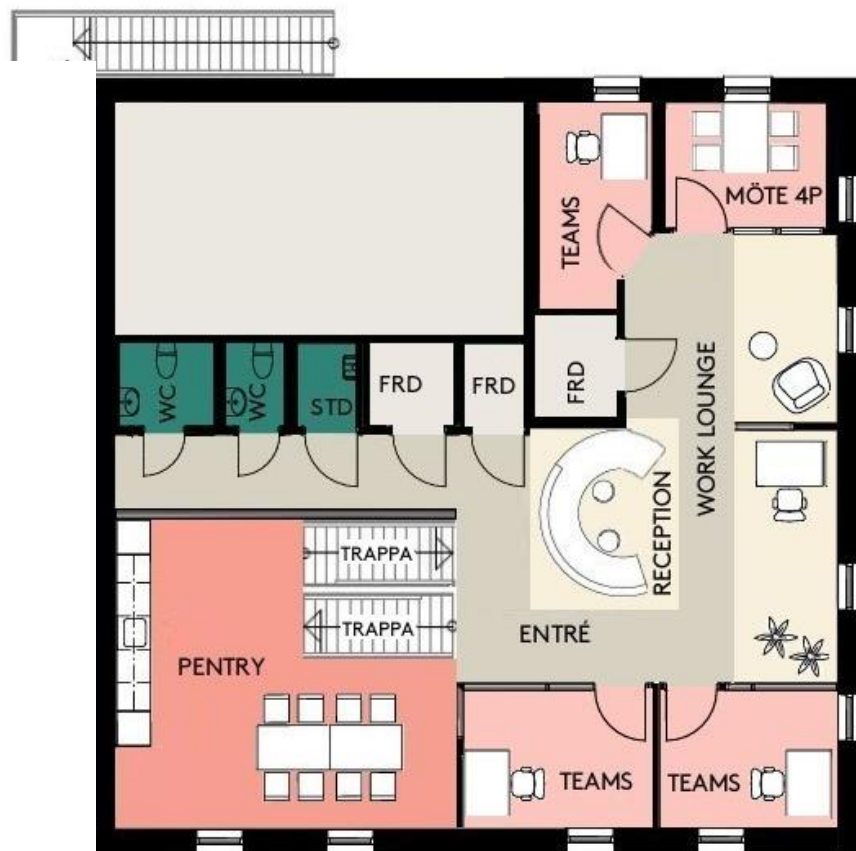
Våning 1: Kontor, mötesrum, wc dusch, städ och pentry.
